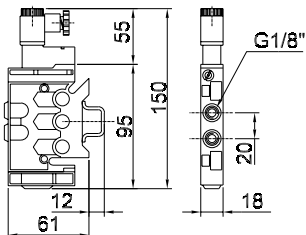
Simples solenóide
