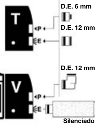
Silenciador
