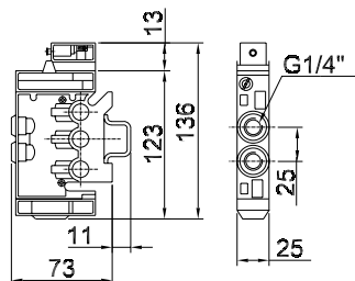
Simples piloto
