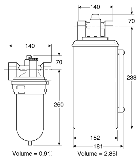
Lubrificador
