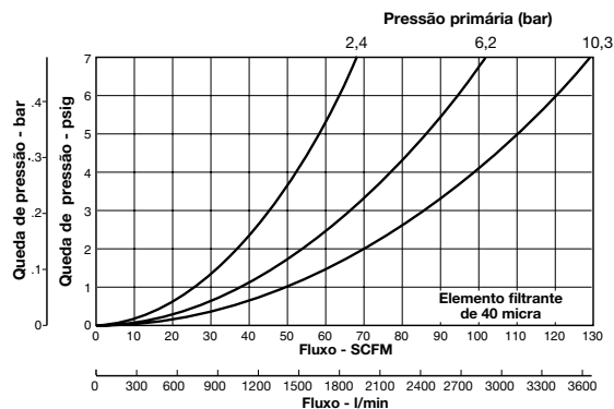
Rosca de 1/2"
