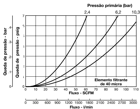
Rosca de 3/8"
