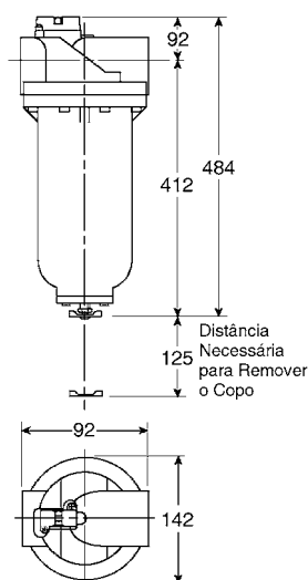
Filtro
