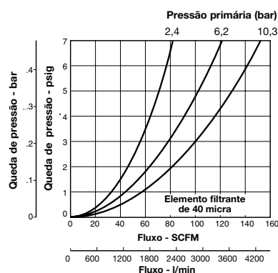
Rosca de 3/8"
